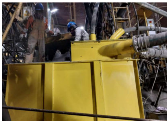
Fabricación y cambio de caja alim OK8
