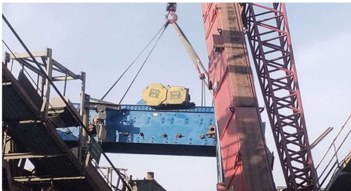
Cambio de la zaranda de 5x16
