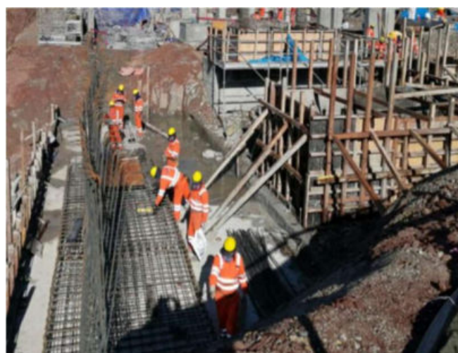
Obras civiles planta de filtrado de relaves Chungar (Parte de la mano de obra)
